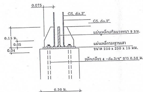
ขยายการติดต่อหลักกับเสา ค.ส.ล.
