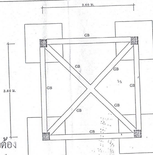
แปลนฐานราก คำนวณคอดิน มาตราส่วน 1 : 50
