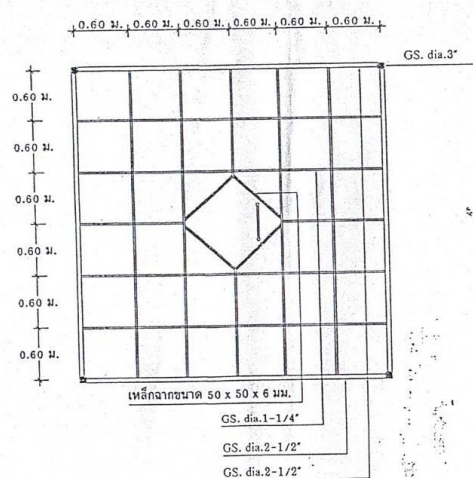
แปลนโครงเหล็กรับดิ่งน้ำในระดับ A มาตราส่วน 1:50
