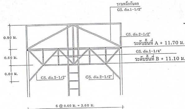
แบบขยายโครงเหล็กรับดิ่งน้ำ มาตราส่วน 1:50
