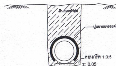
แบบรูปตัดจุดดินวางท่อ
