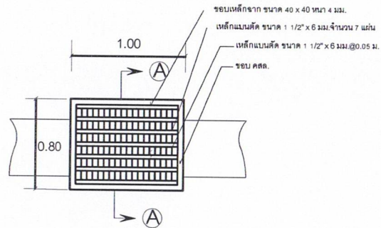
แบบแปลนบ่อพักน้ำ
