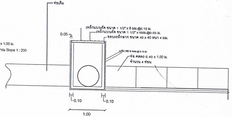
รูปตัดบ่อพักน้ำ จุดที่ 1 - จุดที่ 7
