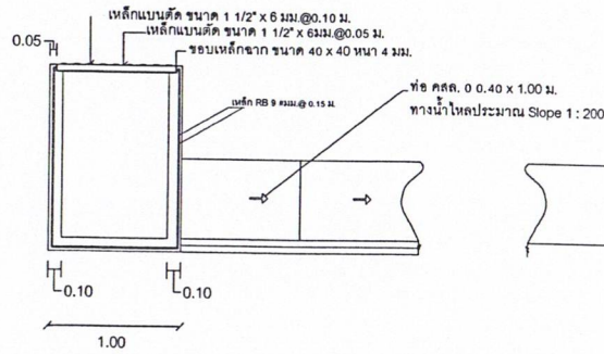
รูปตัดบ่อพักน้ำ จุดที่ 1 - จุดที่ 7
