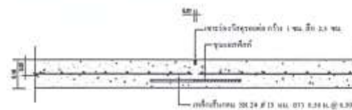
แบบขยาย \Delta CONTRACTION JOINT
