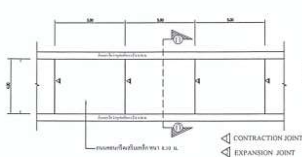
แบบปรับปรุงถนนคอนกรีตเสริมเหล็ก
