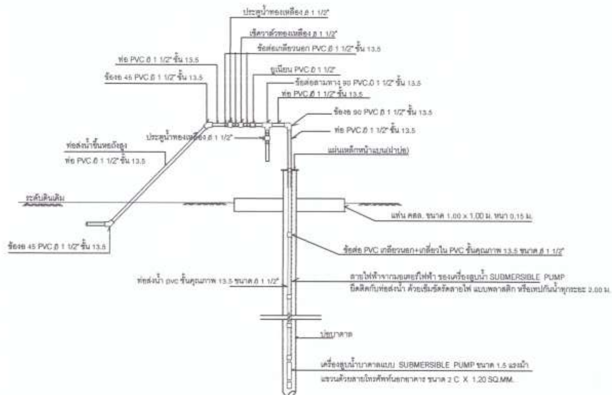
การประสานท่อที่ปากบ่อนบาดาลการติดตั้งเครื่องสูบน้ำบาดาล แบบขั้วเมิลซีเมนต์
