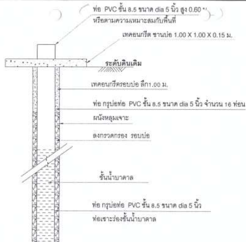
รูปตัดบ่อน้ำบาดาล
