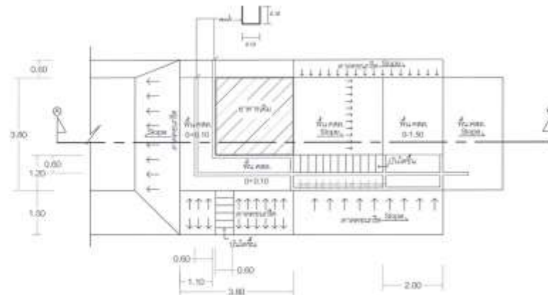
แบบแปลน
