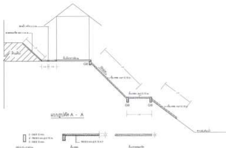
แบบดูดน้ำ GB, พื้น คสล., พื้นลาดคอนกรีต
