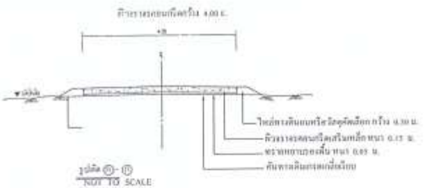
แบบถนบกอนกรีตเสริมเหล็ก
