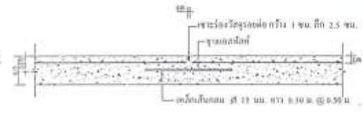
แบบถนบ CONTRACTION JOINT
